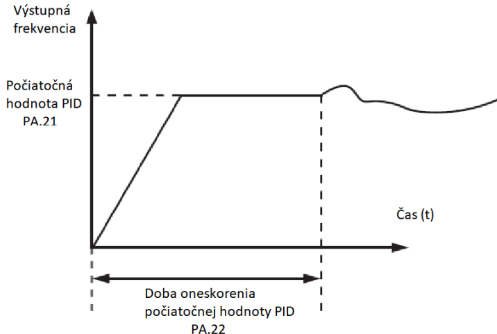
4-25 Funkcie počiatočnej hodnoty PID
